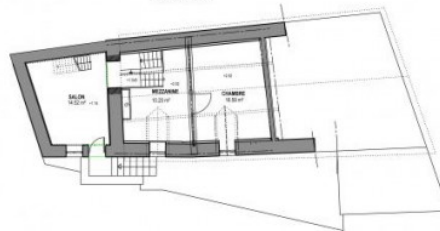
PLAN DU COMBLE
